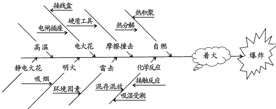
图 3-1 烟花爆竹引爆的因果分析图
